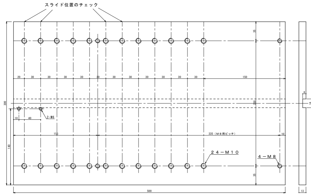
TRFスライドプレート (TRF202, 302, 402 共通) 材料 SS400 300×500×13
