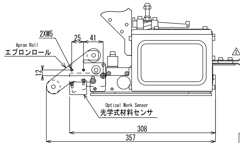
Example of Mounting Optional Products オプション製品取付例
