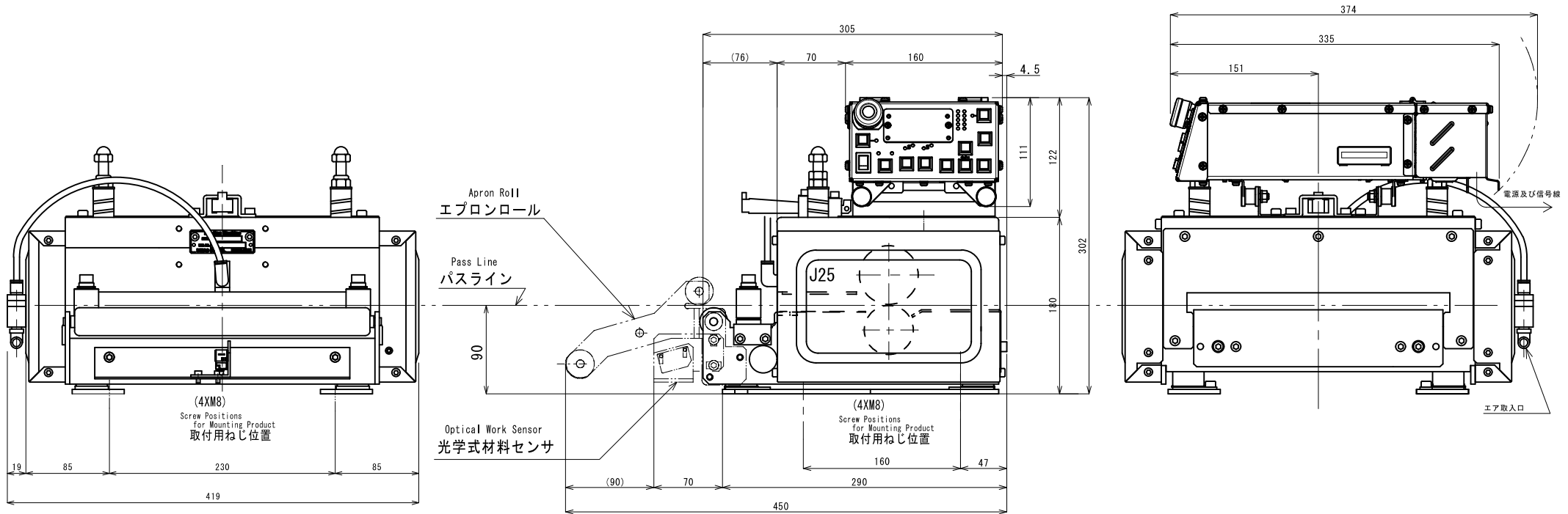
Example of Mounting Optional Products オプション製品取付例
